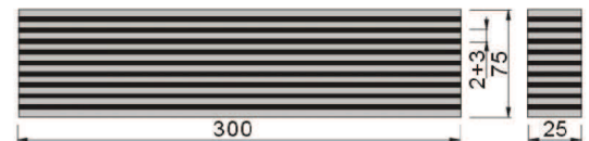
54020-10 HTL-300
