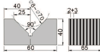
54020-04 HTV-60
