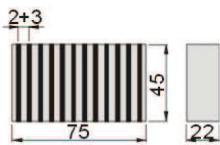
54020-03 HT-75
